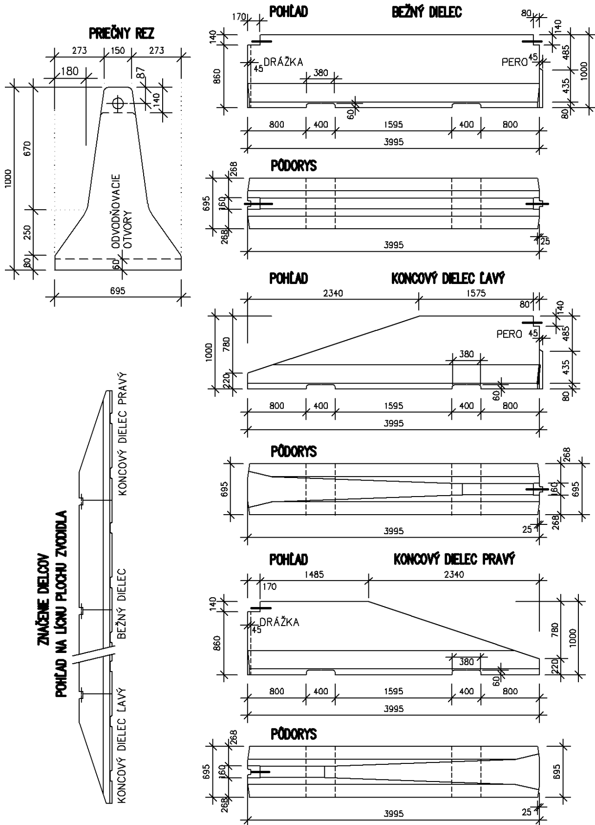
Obrázok 5 – Obojstranné betónové zvodidlo výšky 1 m – bežný a koncový dielc, v (mm)
