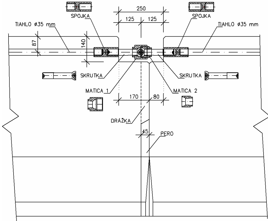
Obrázok 1 – Zámok zvodidiel – spojka, v (mm)
