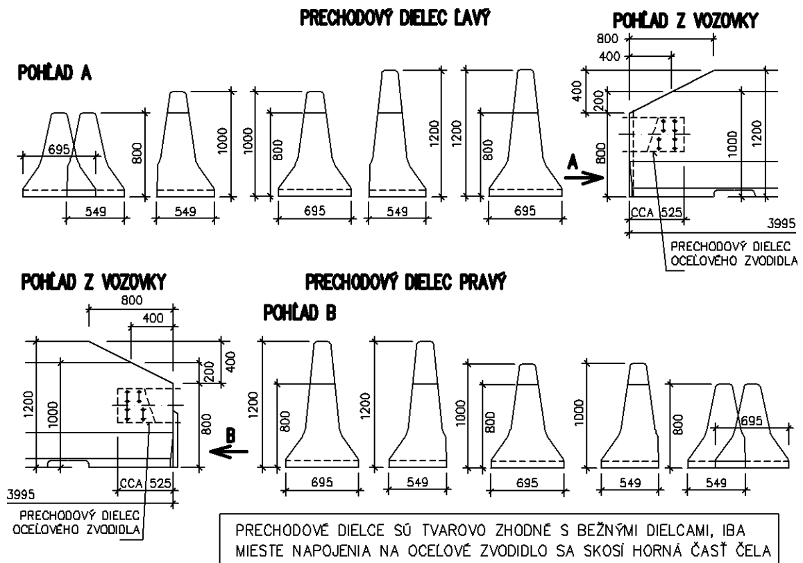
Obrázok 9 – Prechodové dielce na oceľové zvodidlo, v (mm)
