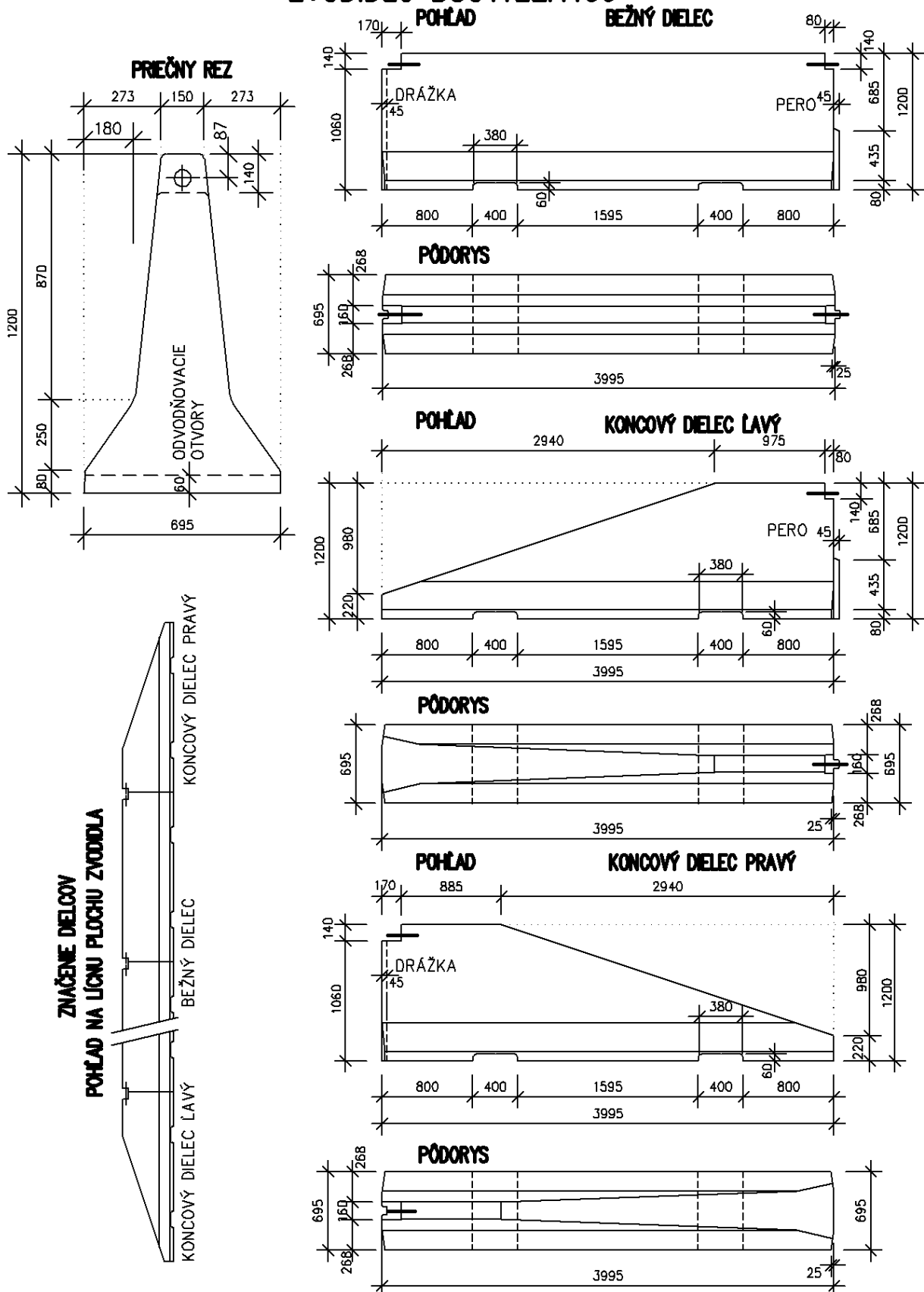
Obrázok 7 – Obojstranné betónové zvodidlo výšky 1,2 m – bežný a koncový dielc, v (mm)
