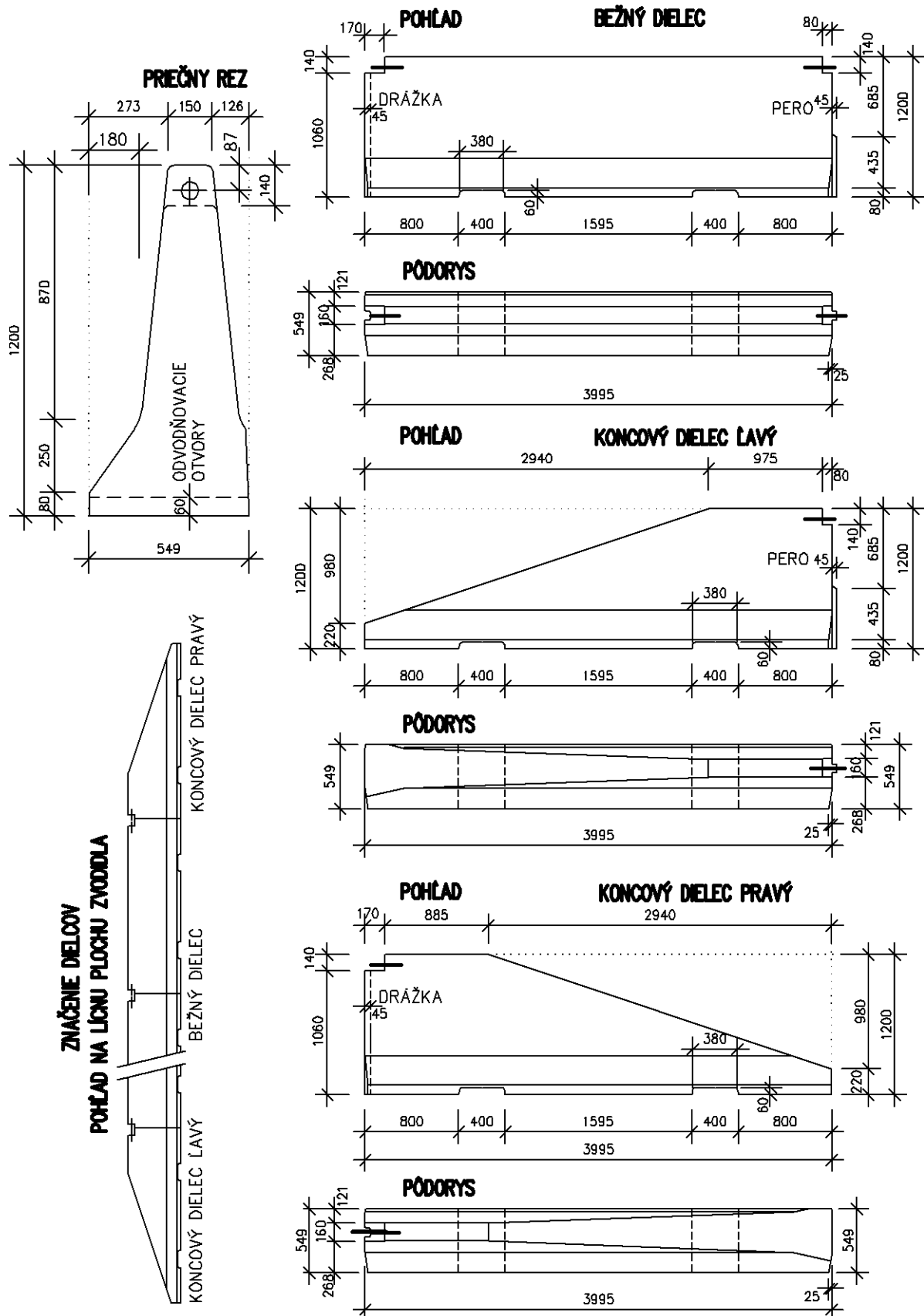
Obrázok 6 – Jednostranné betónové zvodidlo výšky 1,2 m – bežný a koncový dielc, v (mm)
